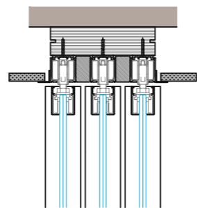
Трехпутный скрытый трек Three ways build-in track
