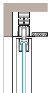
Однопутный скрытый трек вдоль стены Single build-in track against wall
